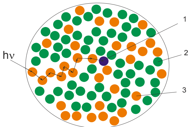
Рис. 28. Схема будови фотосистеми листя рослини (1 – реакційний центр фотосистеми, 2 – молекула хлорофілу, 3 – молекула каротиноїду)
