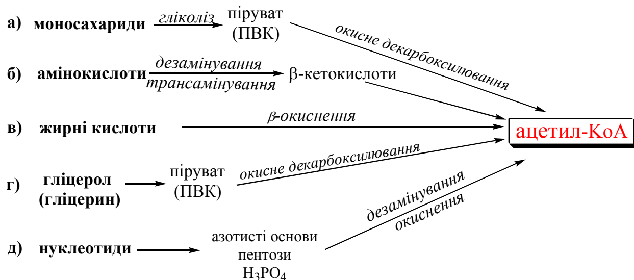
Рис. 4. Друга стадія катаболізму біомолекул
