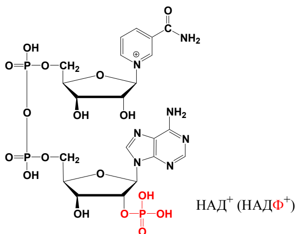
Рис. 8. Структура НАД + (НАДФ + )
