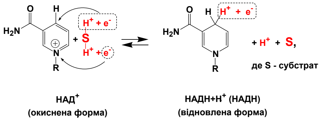
Рис. 9. Утворення відновленої форми НАДН+Н +
