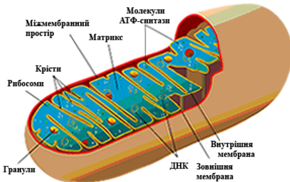
Рис. 6. Будова мітохондрії (Mariana Ruiz Villarreal, 2006)
