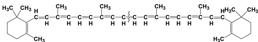
Рис. 27. Будова молекули \beta -каротину
