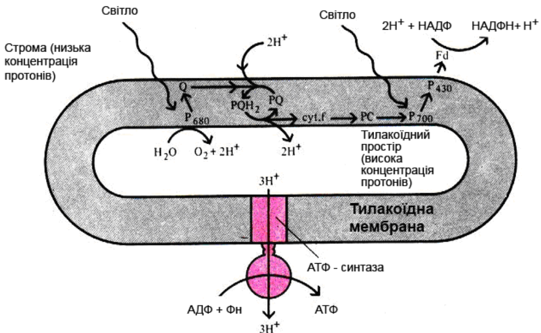
Рис. 32. Розташування компонентів процесів фотосинтезу та фотофосфорилування в тилакоїдах: пігмент \text{P}_{680} – реакційний центр фотосистеми II, Q – кофактор Q (феофітин), \text{PQH}_2 – пластохінон
