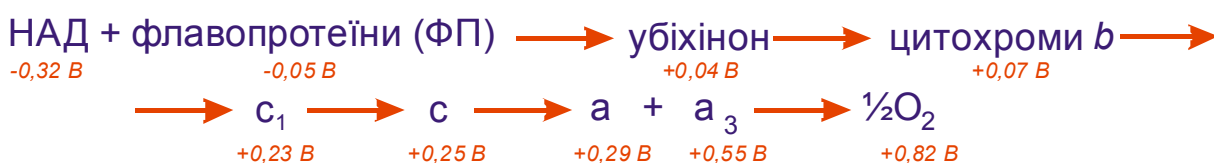
Рис. 16. Зміна значень Ох-Red-потенціалів компонентів дихального ланцюга мітохондрій
