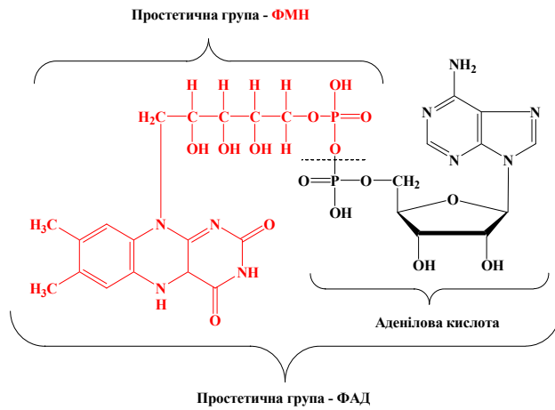
Рис. 10. Структура ФМН, ФАД
