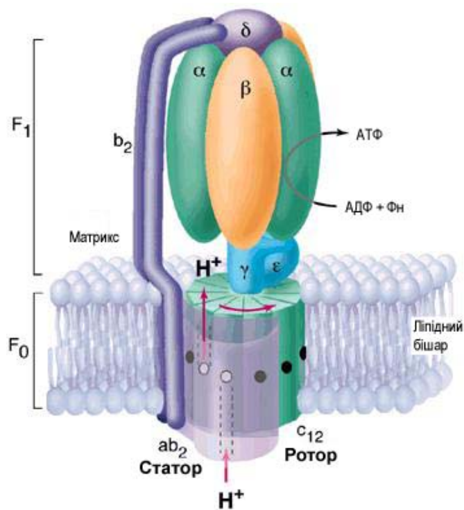
Рис. 19. Структура АТФ-синтази (Pizzo S.V., 2011 зі змінами)
