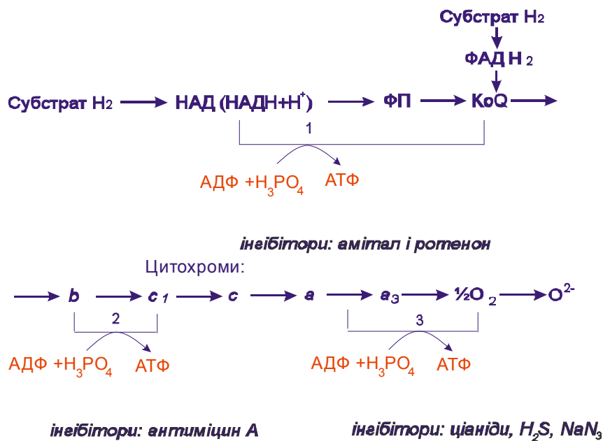
Рис. 17. Локалізація трьох пунктів спряження дихання й фосфорилування в дихальному ланцюзі
