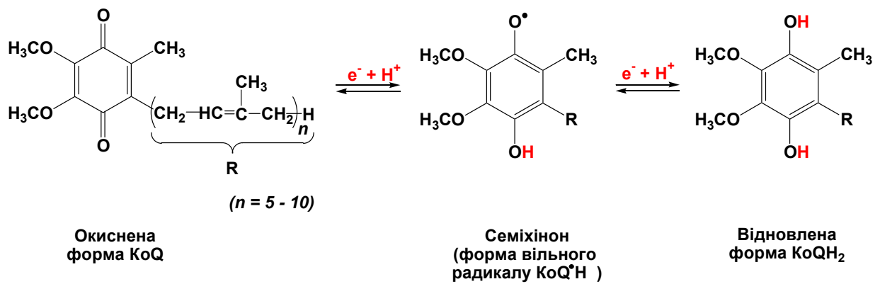
Рис. 12. Убіхінон. Перенос протонів і електронів
