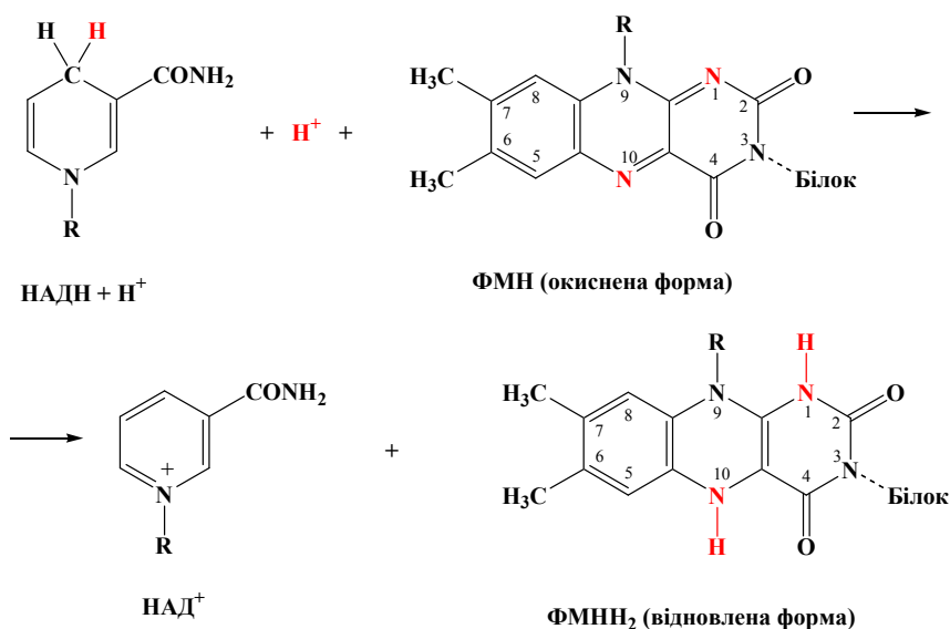
Рис. 11. Утворення відновленої форми ФМН
