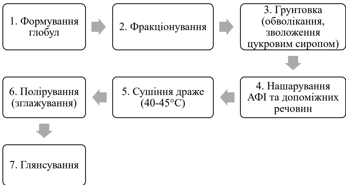
Рис. 4. Основні стадії процесу дражування [джерело: власна розробка]
