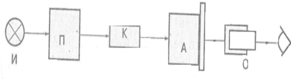
Рис. 15.7 Схема поляриметра
