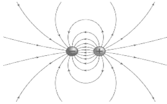
Рис. 10.4 Силві лінії електричного поля, утвореного диполем
