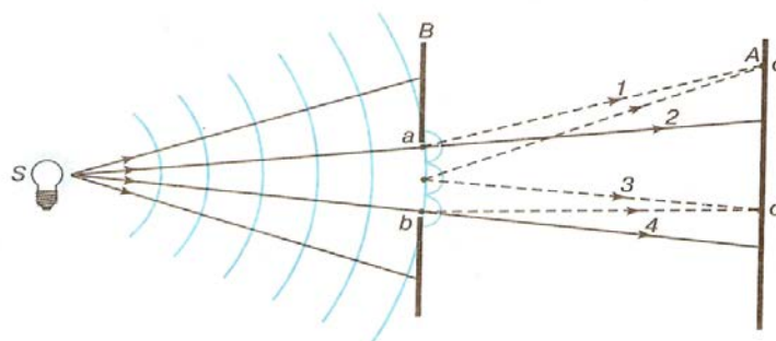
Рис. 15.3 Дифракція світла
