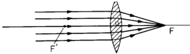
Рис. 14.5 Заломлення променів у збірній лінзі
