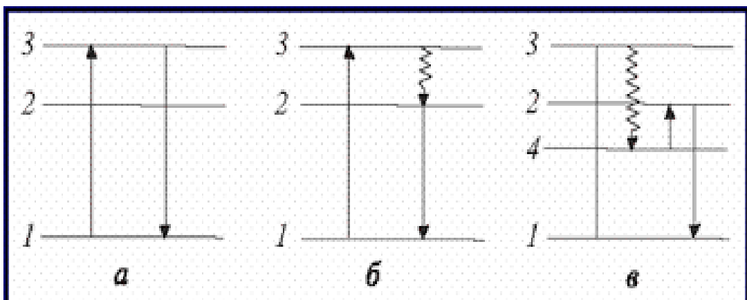
Рис. 19.1 Види люмінесценції
