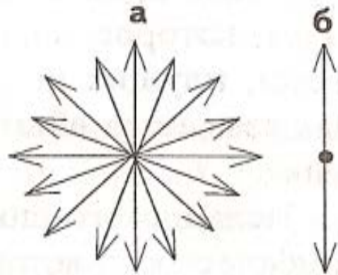
Рис. 15.5 Коливання векторів напруженості електричного поля в природному світлі (а) і в плоскополяризованому світлі (б)
