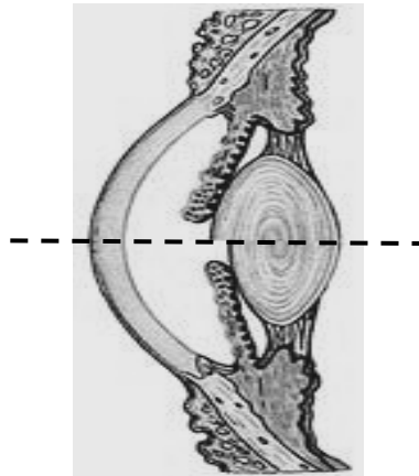
Рис. 17.3 Зміни кривизни кришталика при акомодатції (під пунктиром – його форма при погляді в далеку точку ока, над пунктиром – в ближню)
