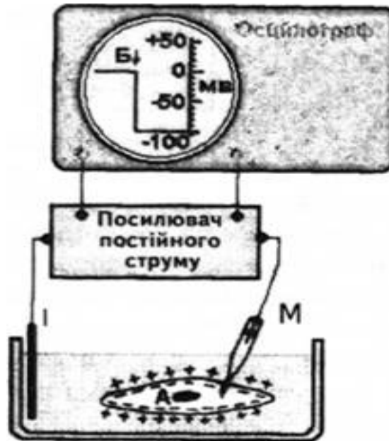
Рис. 8.1 Вимірювання мембранного потенціалу клітини: I - референтний електрод, M – мікроелектрод http://pidruchniki.com/1628041459762/meditsina/fiziologiya_nervovogo_volokna
