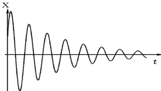
Рис. 1.2 Графік згасаючих гармонічних коливань
