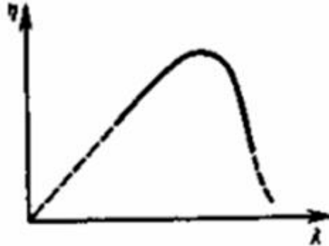
Рис. 1.10. Спектр випромінювання
