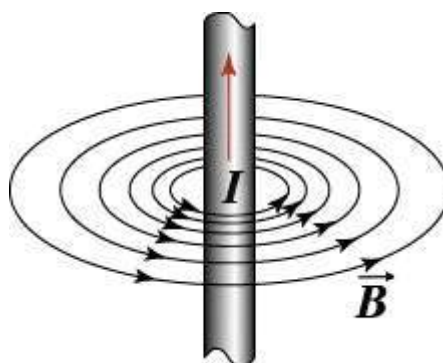
Рис. 12.1 Силві лінії магнітного поля
